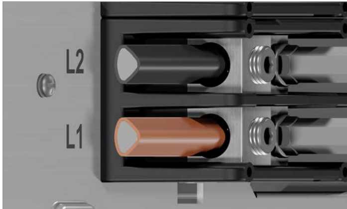
Fig. 7.12 : Emplacement correct des câbles en aluminium sectoriels (2)
