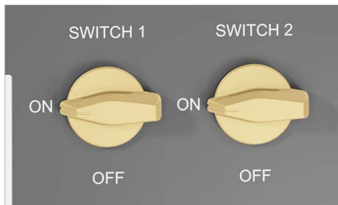
Fig. 4.12 : Coupe-circuits DC tous deux dans la position ON = la connexion aux modules photovoltaïques est fermée
