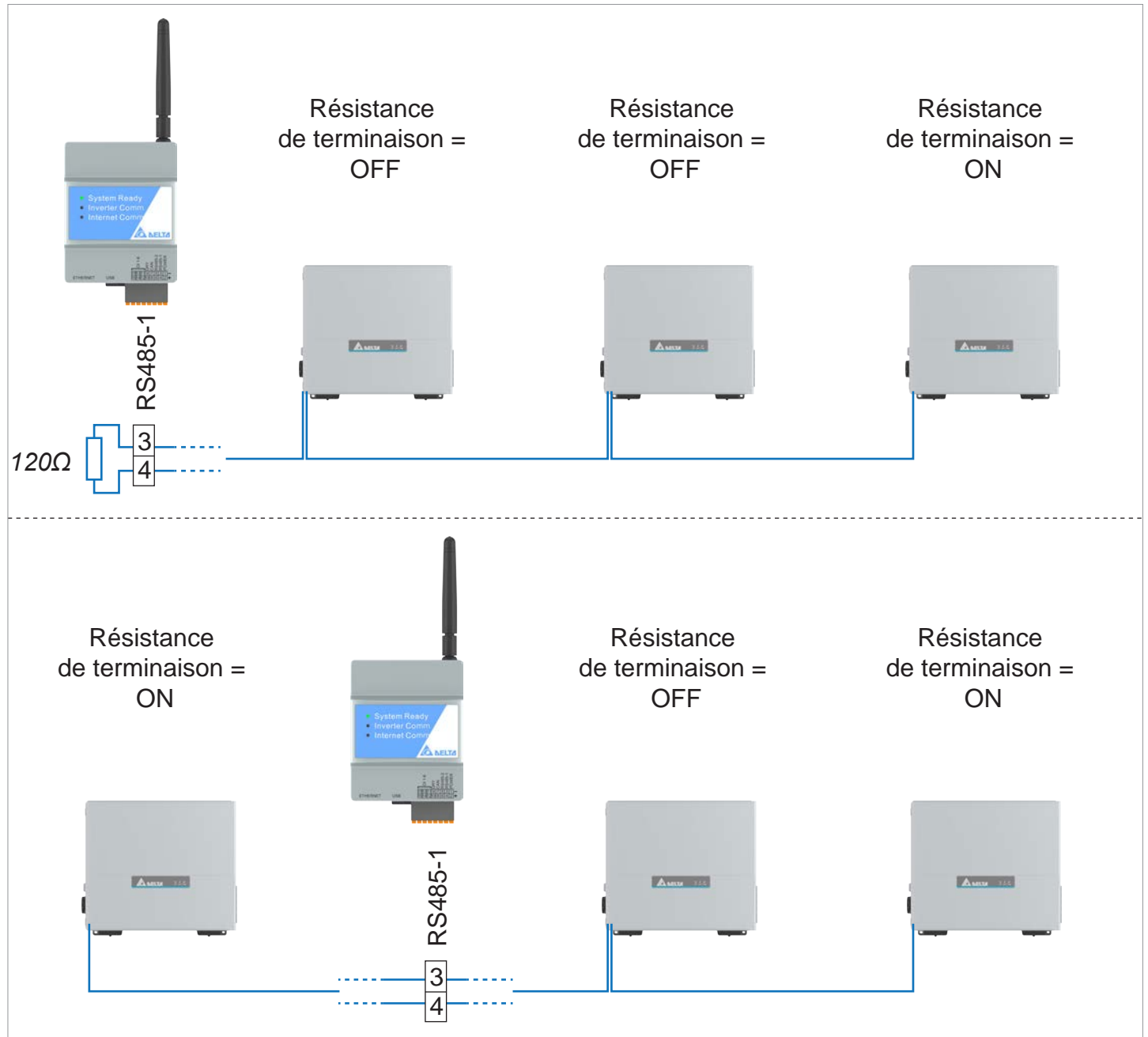
Fig. 7.4 : Schéma de raccordement du RS485 pour un collecteur de données DC1 avec plusieurs onduleurs
