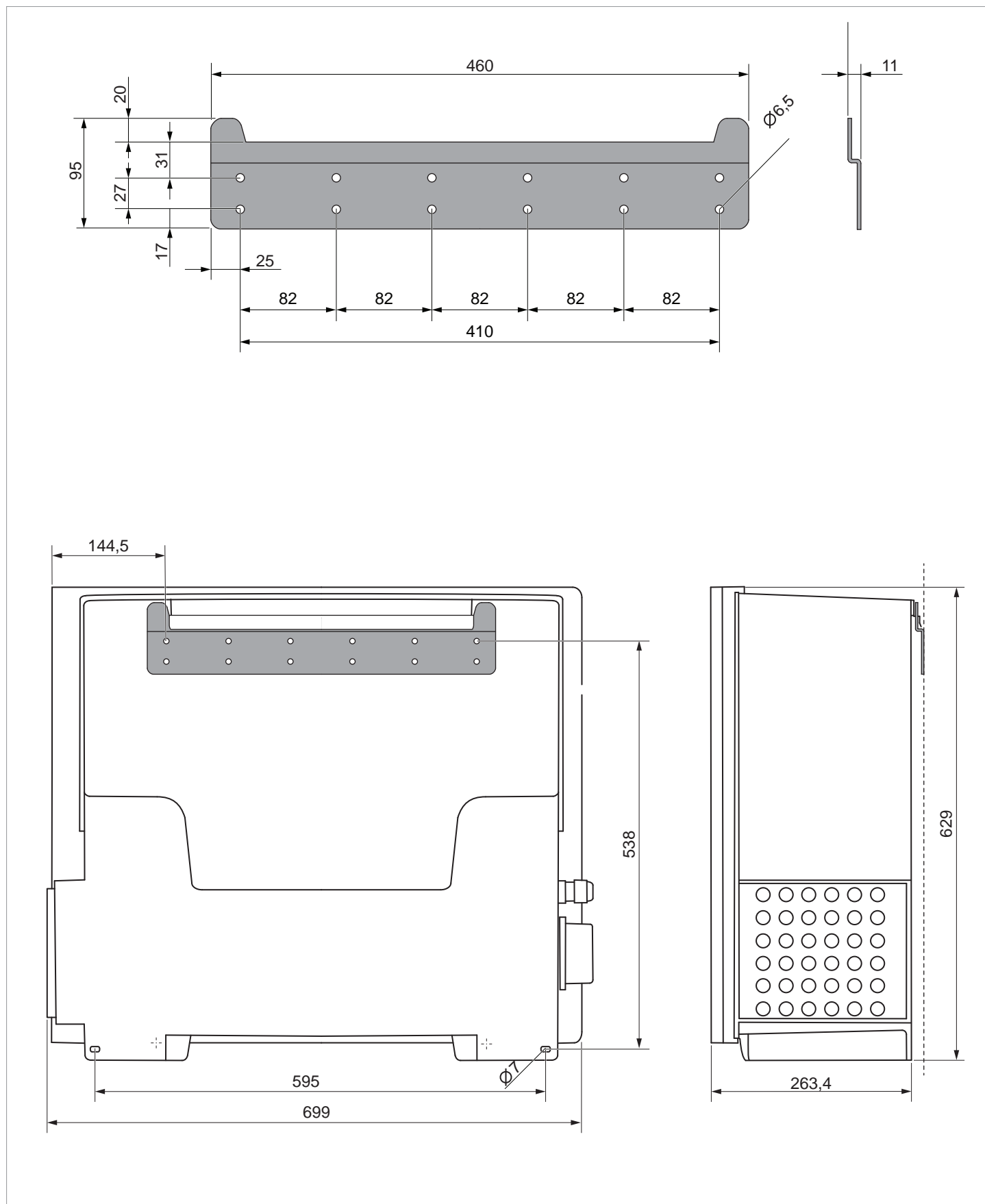
Fig. 5.11 : Onduleur avec plaque de montage, dimensions sans antennes (indications en mm)
