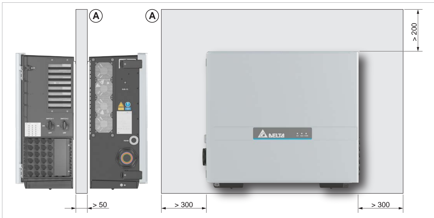
Fig. 5.6 : Espacements de montage et circulation de l'air, variante 3 (indications en mm)
