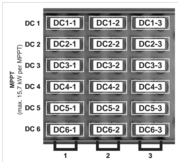
Fig. 5.23 : Disposition des entrées DC sur le panneau de connexion DC
