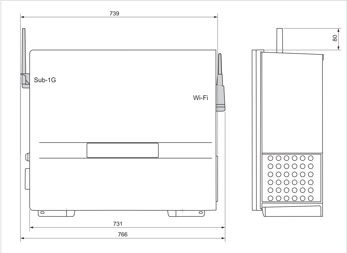
Fig. 5.12 : Onduleur, dimensions avec antennes (indications en mm)
