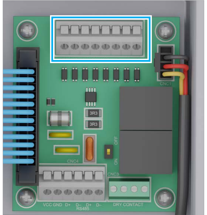
Fig. 5.30 : Bornier avec entrées numériques
