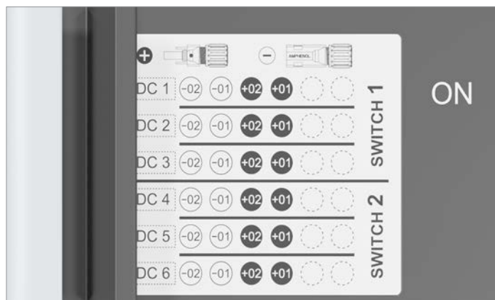
Fig. 4.9 : Étiquette d'affectation des différents connecteurs DC
