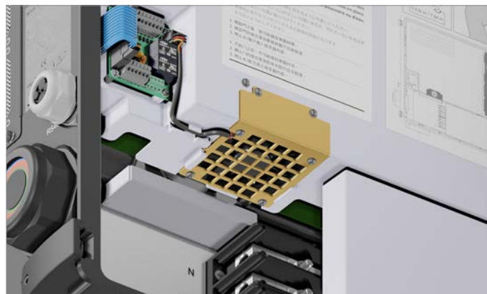
Fig. 4.21 : Ventilateur interne 1
