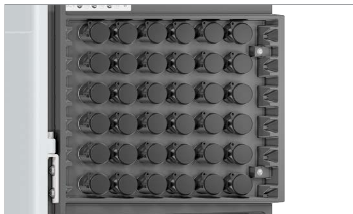
Fig. 4.8 : Panneau de connexion DC sans plaque de recouvrement DC
