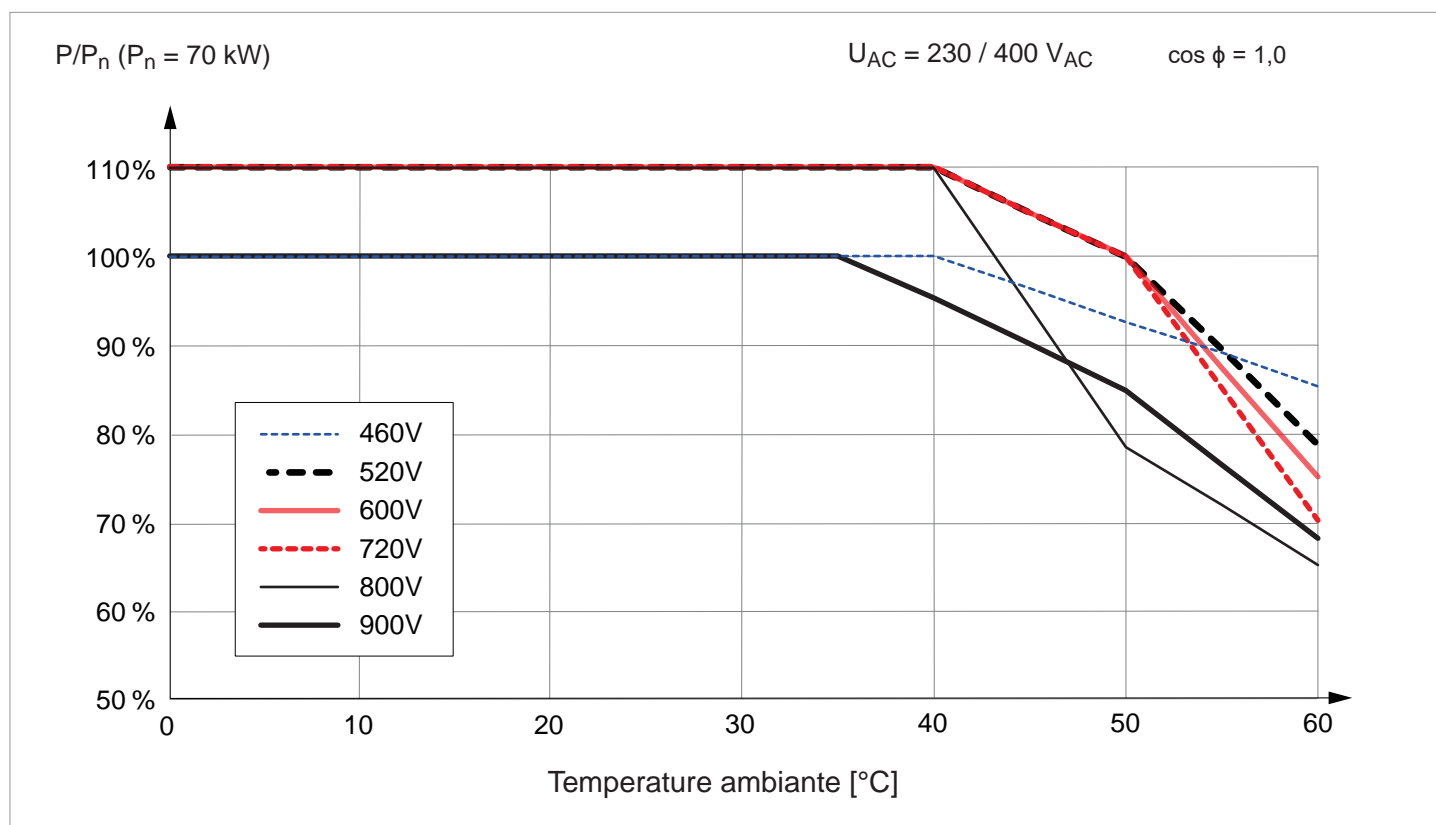
Fig. 5.8 : Courbe caractéristique « Régulation de puissance active en fonction de la température ambiante, \cos \phi = 1,0 ; tension AC = 230 / 400 V AC »
