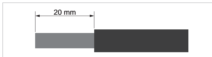
Fig. 7.10 : Longueur d'isolation pour câbles AC
