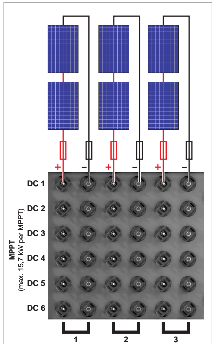
Fig. 5.26 : Raccordement de 3 chaînes de modules par entrée DC (= régulateur MPP) : fusibles de chaîne recommandés
