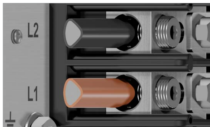
Fig. 5.20 : Emplacement correct des câbles en aluminium sectoriels (2)
