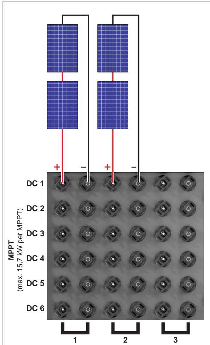
Fig. 5.25 : Raccordement de 1 ou 2 chaînes de modules par entrée DC (= régulateur MPP) : aucun fusible de chaîne nécessaire
