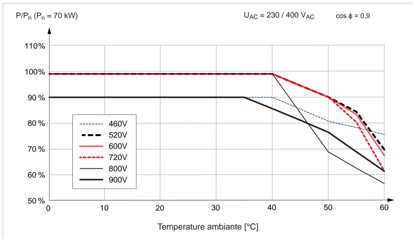
Fig. 5.7 : Courbe caractéristique « Régulation de puissance active en fonction de la température ambiante, \cos \phi = 0,90 ; tension AC = 230 / 400 V AC »
