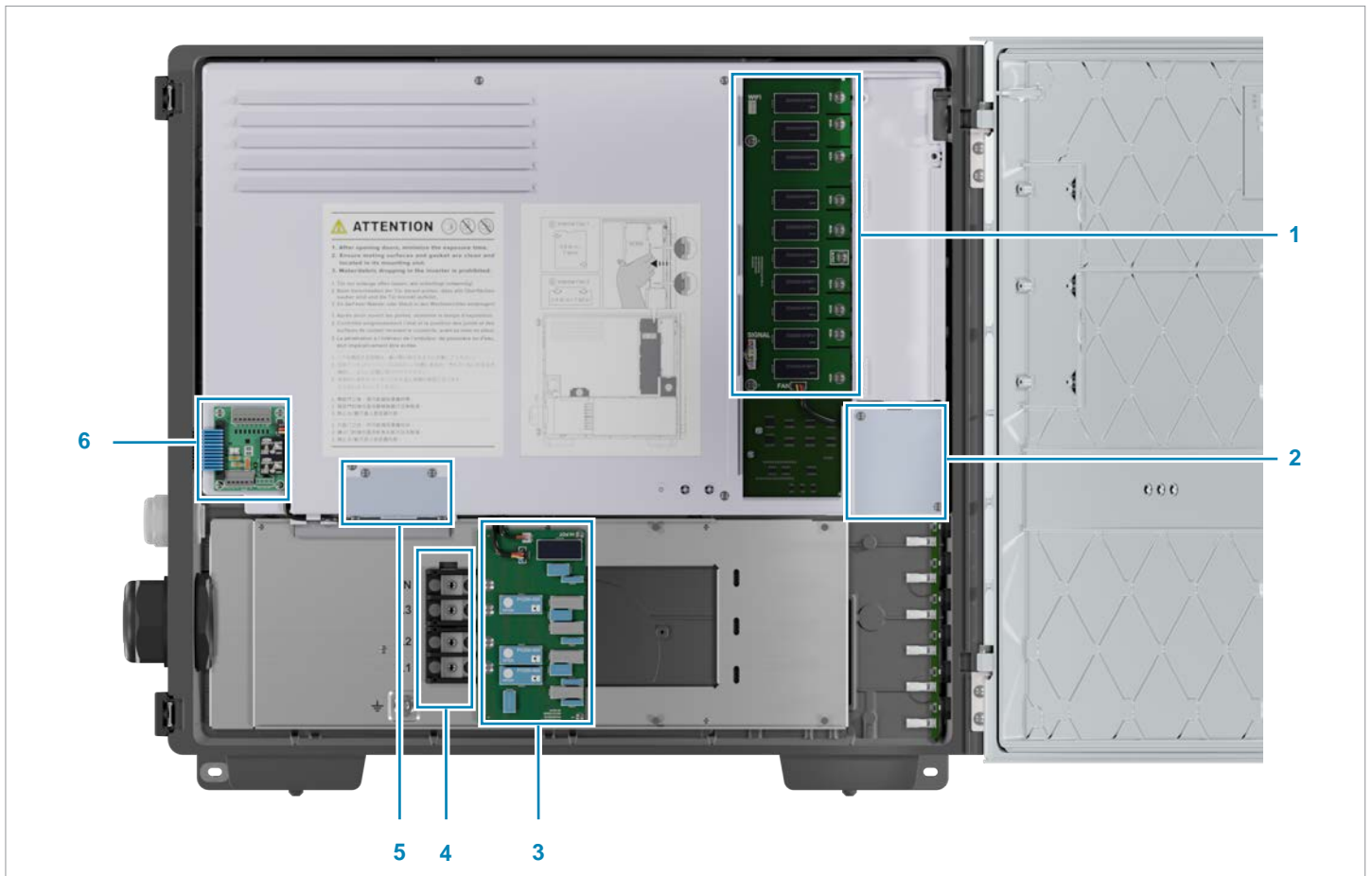
Fig. 4.2 : Vue d'ensemble des composants internes lorsque le couvercle de protection est retiré
