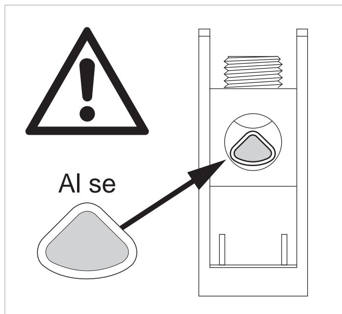
Fig. 5.19 : Emplacement correct des câbles en aluminium sectoriels (1)
