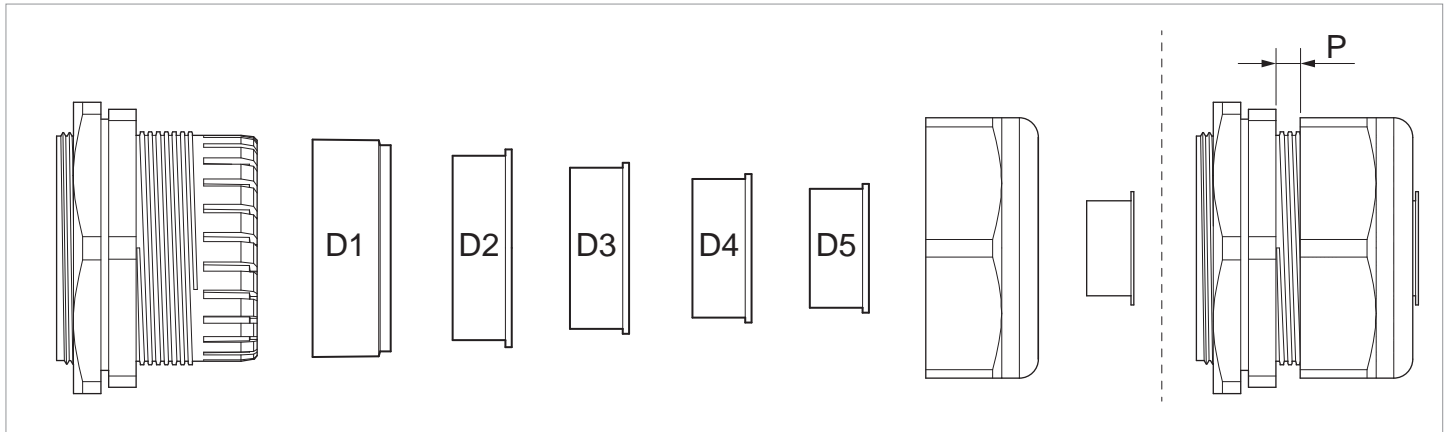
Fig. 7.15 : Utilisation des composants du presse-étoupe AC en fonction du diamètre des câbles
