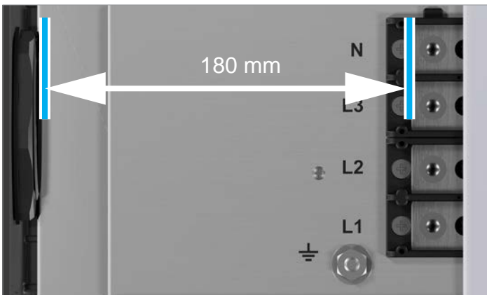
Fig. 5.17 : Espace libre pour le câblage sur le bornier AC
