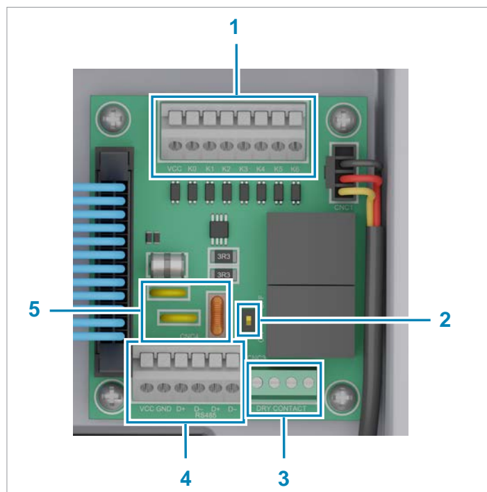
Fig. 4.15 : Composants de la carte de communication
