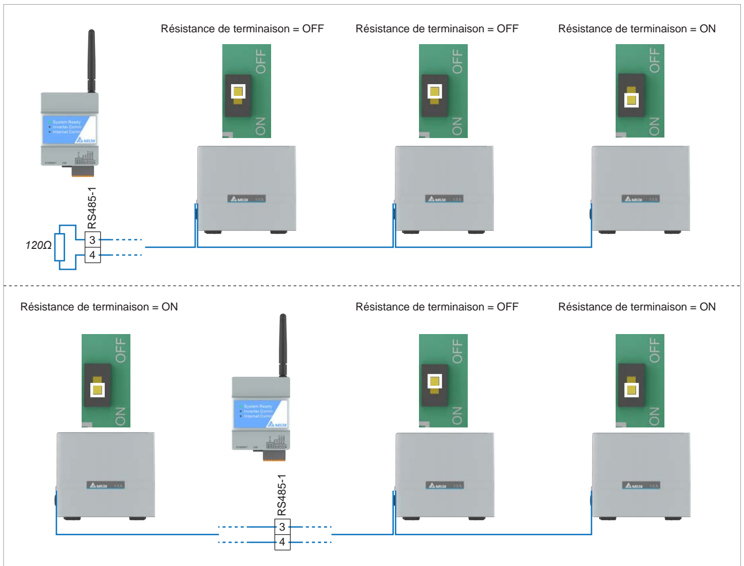
Fig. 5.29 : Schéma de raccordement du RS485 pour un collecteur de données DC1 avec plusieurs onduleurs
