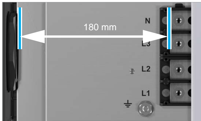
Fig. 7.8 : Espace libre pour le câblage sur le bornier AC
