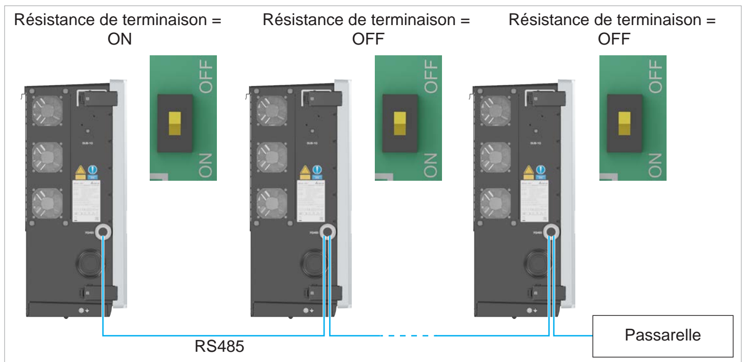
Fig. 7.3 : Schéma de raccordement du RS485 pour plusieurs onduleurs
