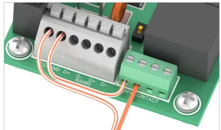
Fig. 7.6 : Exemple de raccordement : raccordement de 1 dispositif d'alarme externe avec alimentation en tension interne de 12 V DC aux contacts sans potentiel
