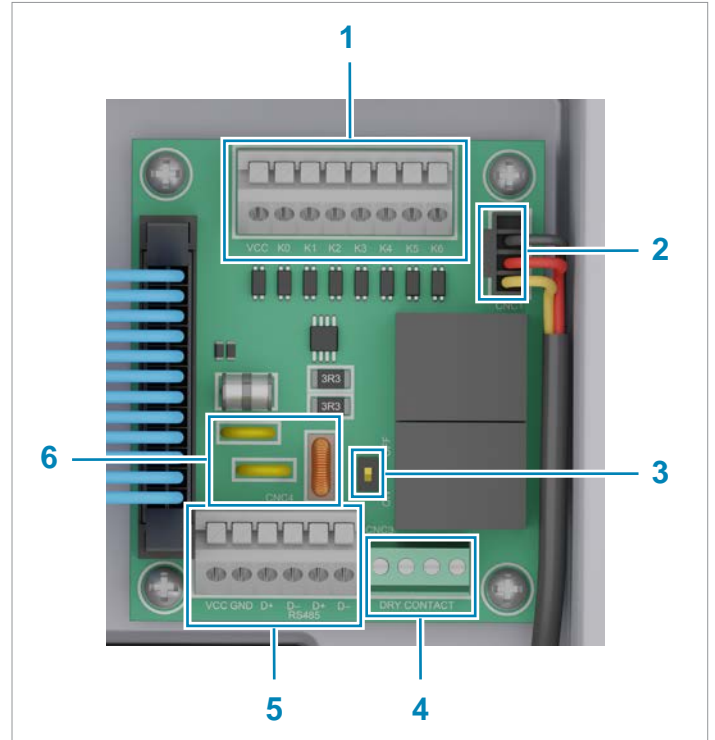
Fig. 5.28 : Composants de la carte de communication
