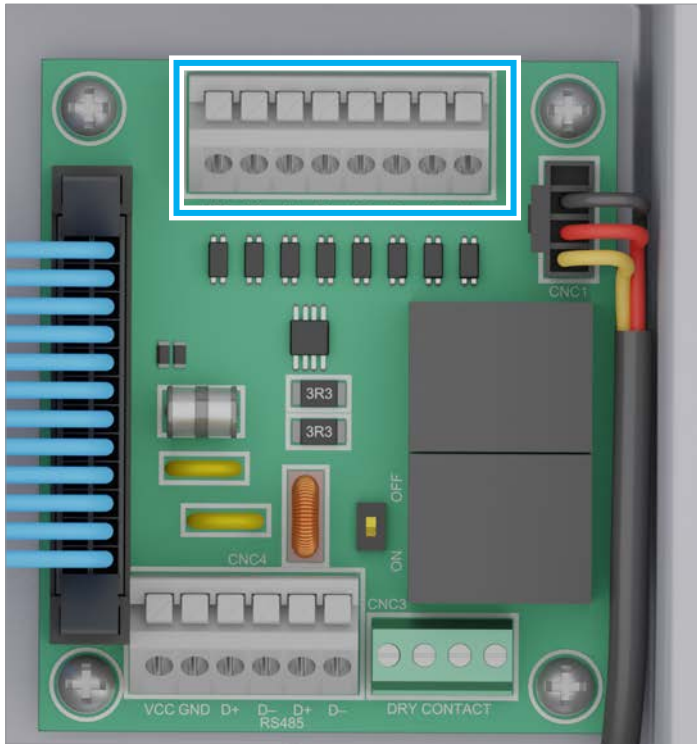
Fig. 5.31 : Bornier avec entrées numériques
