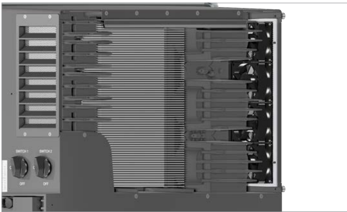
Fig. 4.24 : Dissipateur thermique interne avec plaque de recouvrement arrière retirée
