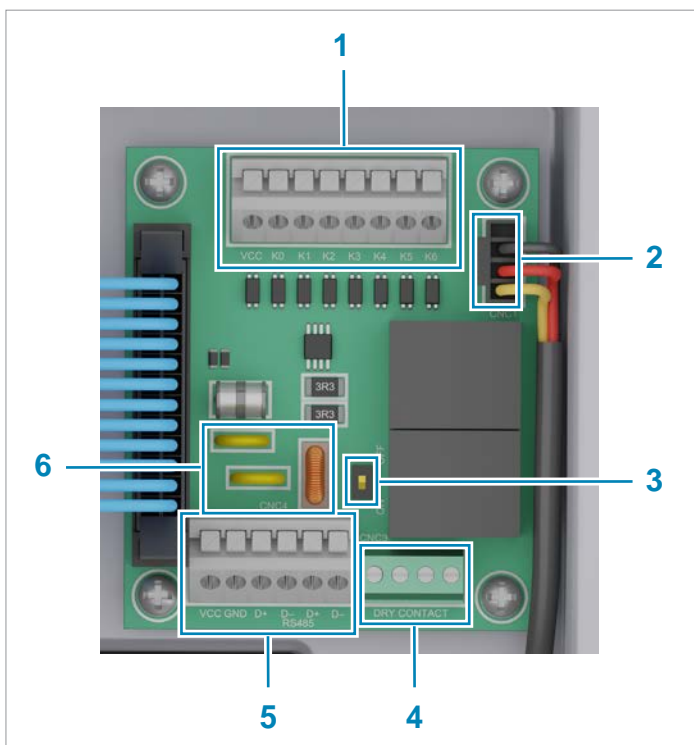
Fig. 7.2 : Composants de la carte de communication
