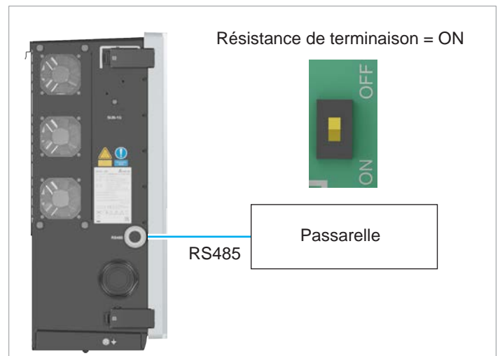
Fig. 7.2 : Schéma de raccordement du RS485 pour un seul onduleur
