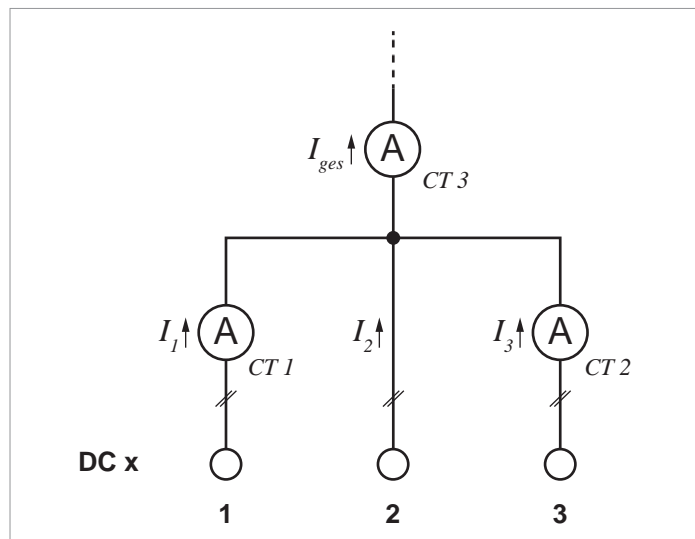
Fig. 5.24 : Disposition des capteurs de courant d'une entrée DC
