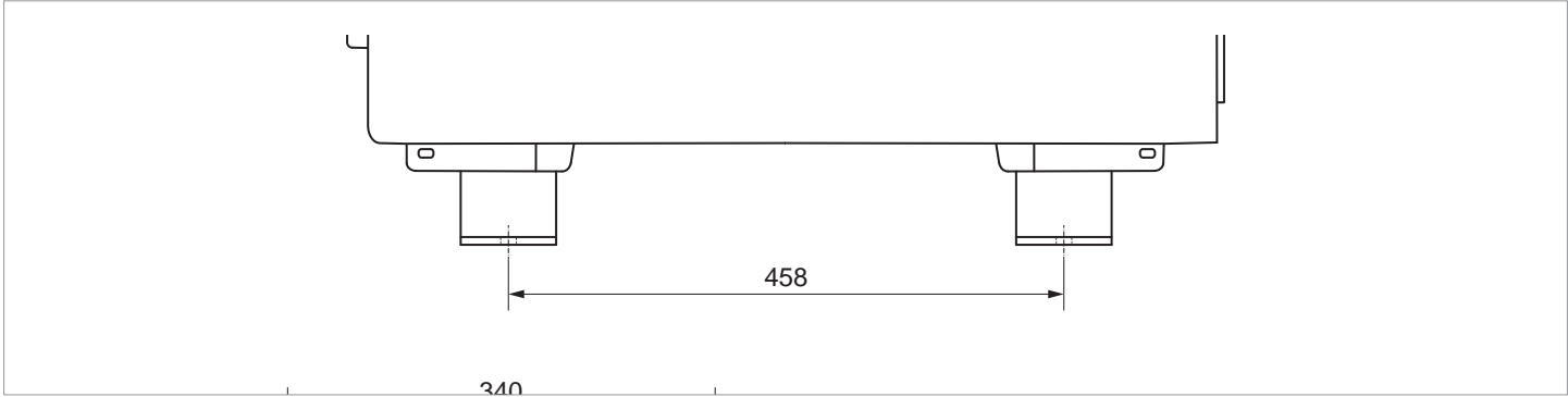
Fig. 5.13 : Pieds pour montage au sol. Dimensions (données en mm)
