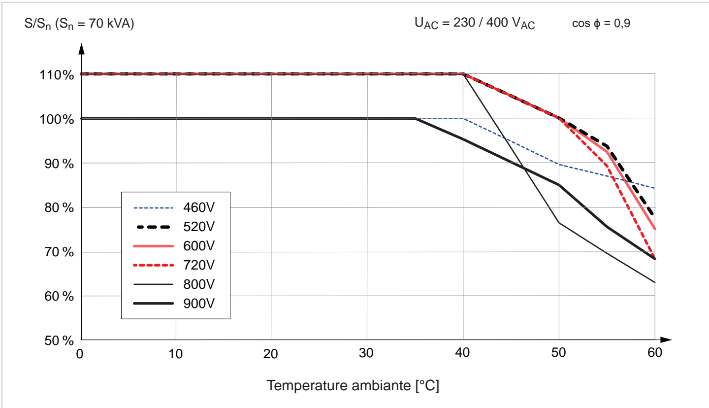
Fig. 5.9 : Courbe caractéristique « Régulation de puissance apparente en fonction de la température ambiante, \cos \phi = 0,90 ; tension AC = 230 / 400 V AC »
